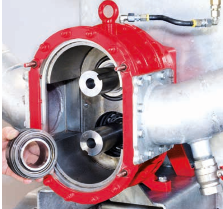
Quality-Cartridge-Dichtung
